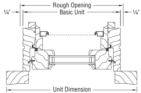
JAMB SECTION
