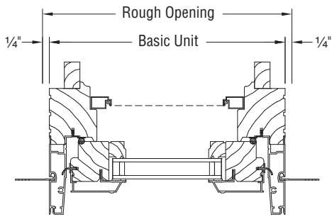
JAMB SECTION
