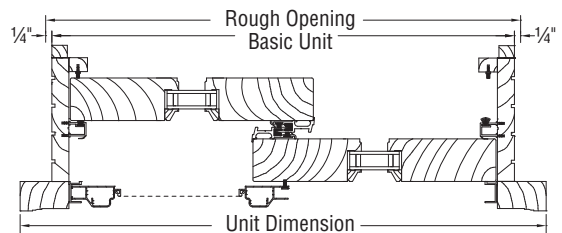
JAMB SECTION
