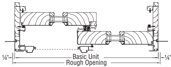
JAMB SECTION
