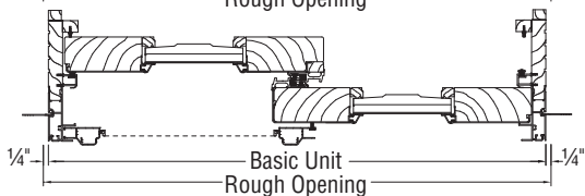
JAMB SECTION
