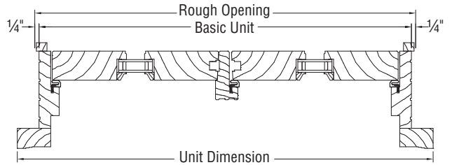
JAMB SECTION
