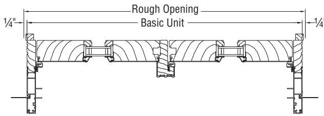
JAMB SECTION
