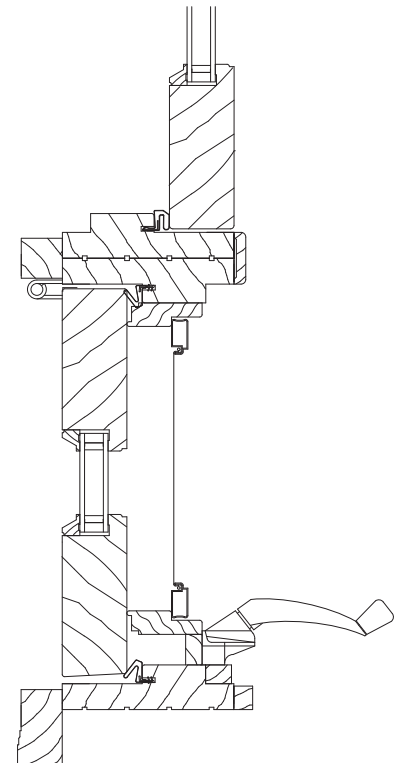
Jamb mullered to CFOD JAMB SECTION
