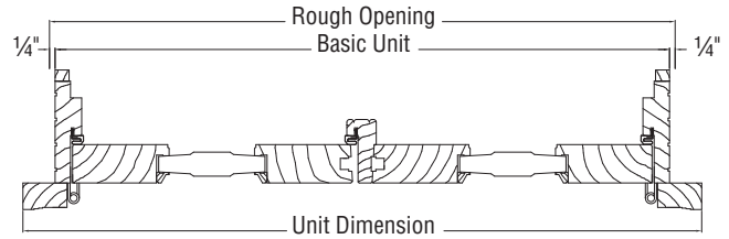
JAMB SECTION
