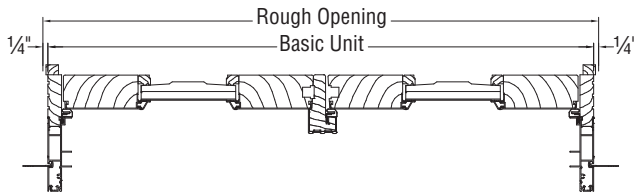
JAMB SECTION
