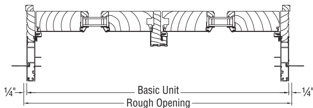
JAMB SECTION
