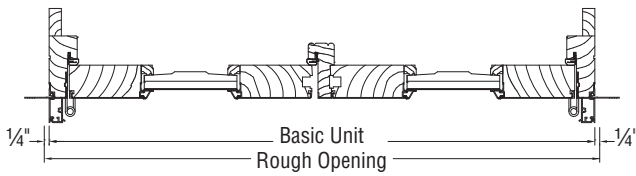
JAMB SECTION
