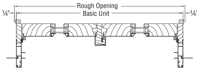
JAMB SECTION
