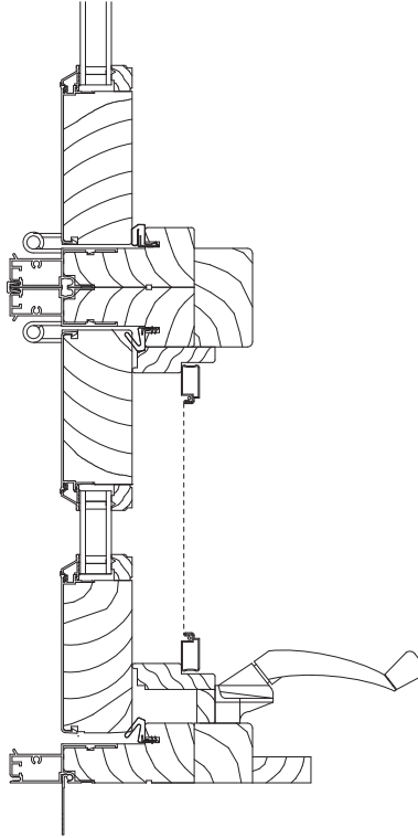
Jamb mullered to CFOD JAMB SECTION
