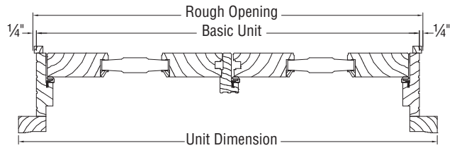
JAMB SECTION
