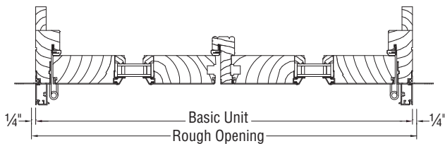
JAMB SECTION
