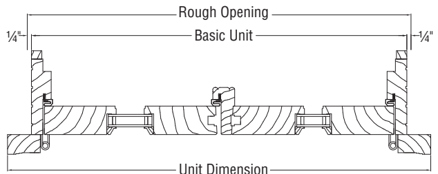
JAMB SECTION
