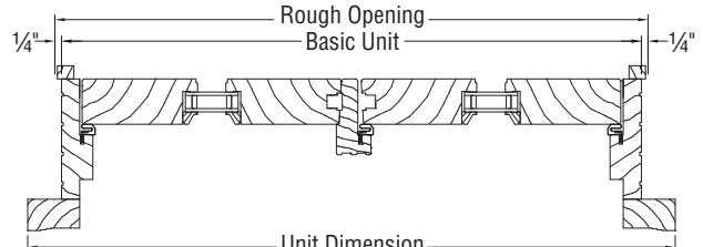
JAMB SECTION
