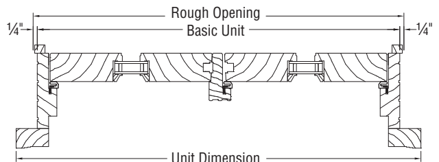
JAMB SECTION
