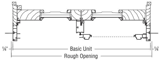
JAMB SECTION
