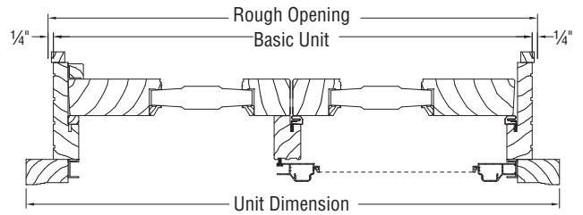
JAMB SECTION
